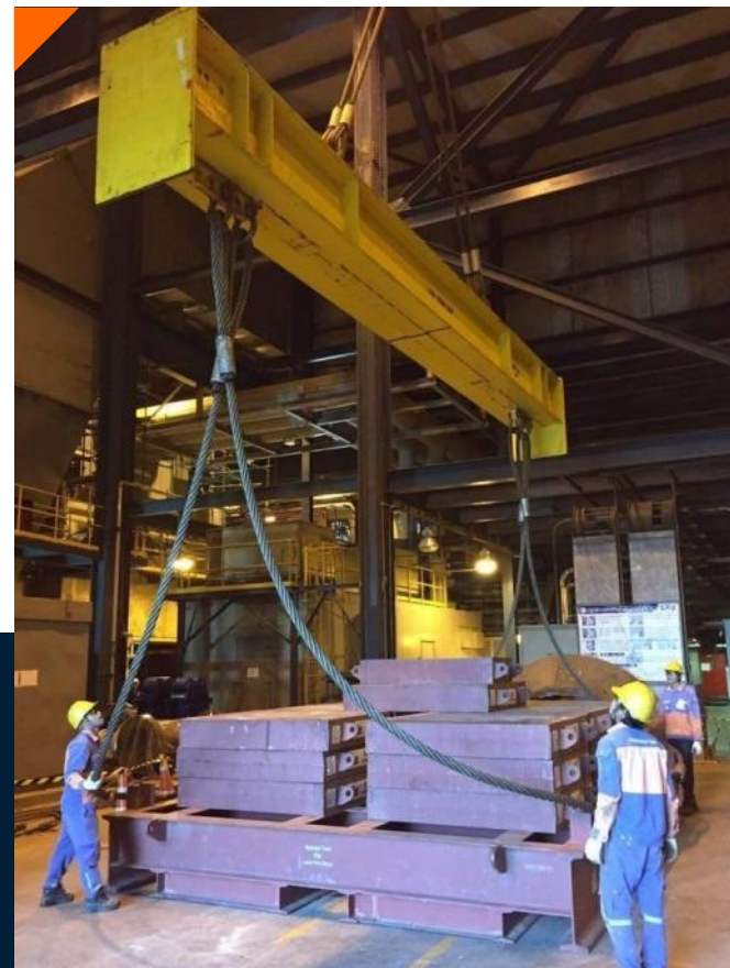
ทดสอบด้วยน้ำหนัก ก้อนเหล็ก
